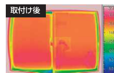
外窓+内窓(インプラス) (単板ガラス3mm+単板ガラス3mm)
